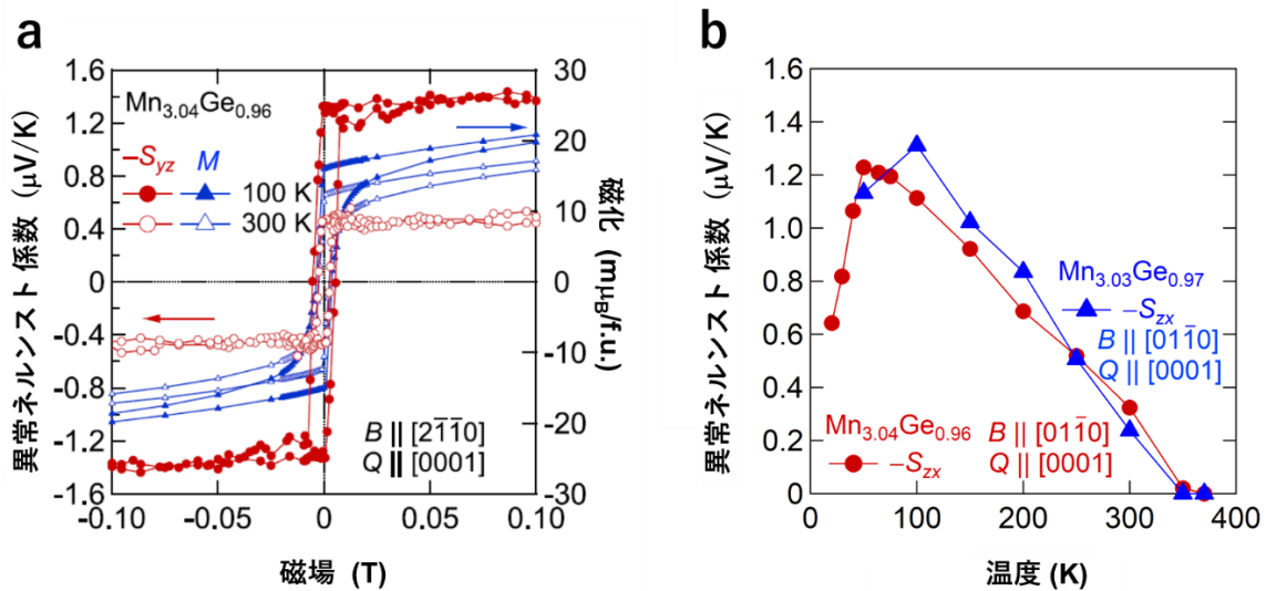
図 2 : (a) \text{Mn}_3\text{Ge} におけるネルンスト係数と磁化の温度依存性。ゼロ磁場でもネルンスト効果がのこるため異常ネルンスト効果を示します。(b) ゼロ磁場での異常ネルンスト効果の温度依存性。温度 100 K にてネルンスト係数が最大値を示します。
