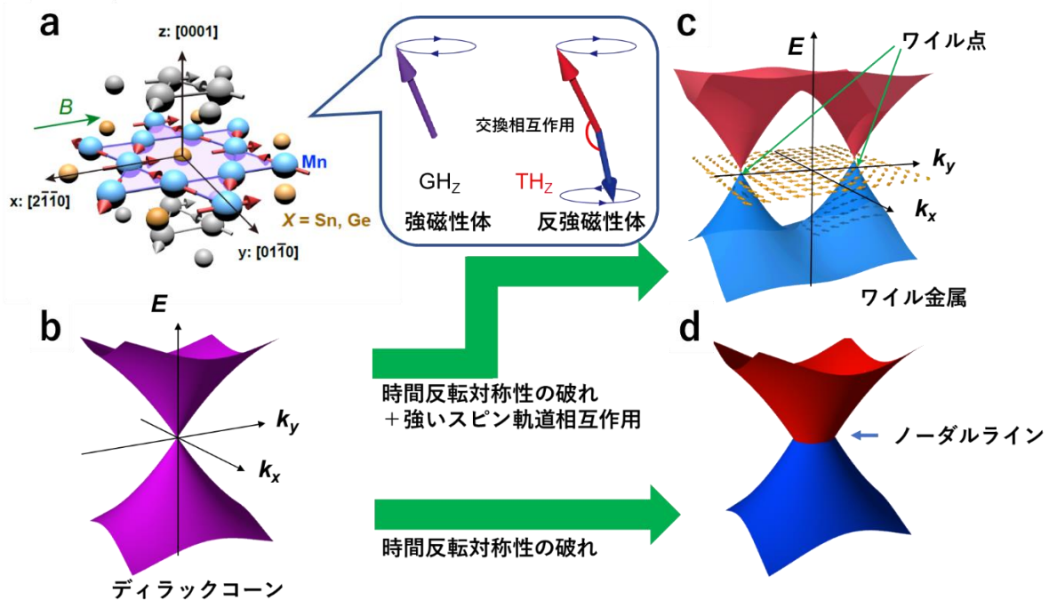
図 1：反強磁性体 Mn_3Ge のワイル粒子生成の概念図。(a) 反強磁性体 Mn_3Ge の実空間での結晶構造と磁場中での磁気構造。 z = 0 面と z = 1/2 面の二層を持つカゴメ格子構造と呼ばれる三角形ベースの結晶構造。磁場 B \parallel [2\bar{1}\bar{1}0] にかけた場合の逆スピン三角構造と呼ばれる Mn (マンガン) スピンの磁気構造の様子。反強磁性体における反強磁性磁気共鳴周波数は交換結合に起因する交換磁場に比例するため、強磁性体に比べて圧倒的に高くなり、テラヘルツ帯の高速動作が可能。(b) 運動量空間でのディラックコーンが対称点にあった際、(c) 磁性体の時間反転の破れによりノーダルラインが現れます。さらに強いスピン軌道相互作用が現れることで、(d) 2点を残したギャップが開くことで運動量空間内に正負のワイル点を持つワイル金属状態が生成されます。
