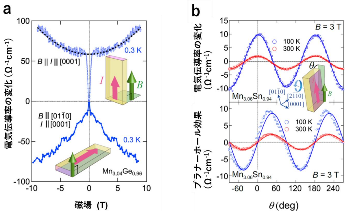
図 3 : (a) 反強磁性体 \text{Mn}_3\text{Ge} の電気伝導率の磁場変化。磁場 B が電流 I と垂直の場合には、正の磁気抵抗(負の電気伝導率)を示すのに対して、磁場と電流が平行の際に負の磁気抵抗(正の電気伝導率)が現れます。これは磁場と電流が平行の際に、磁場の増加ともなう正負のワイル点間のチャージポンピングにより、電気抵抗の減少が見られるカイラル異常と呼ばれる現象で、ワイル粒子が生成された際に現れる特異な効果と考えられています。(b) 電気伝導率と
