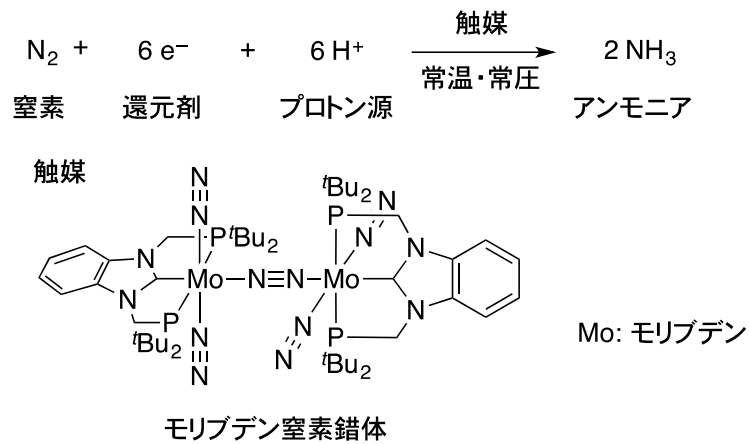
図2. モリブデン窒素錯体による窒素ガスからのアンモニア合成
