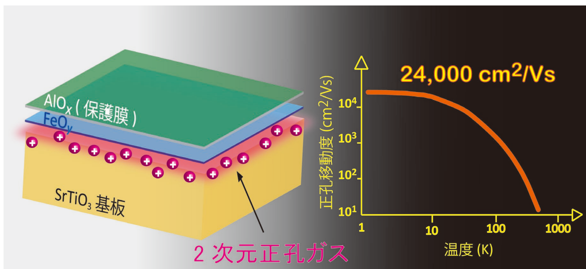
図1 研究グループが作製した試料の構造 (左) と移動度の温度依存性 (右)。 \text{SrTiO}_3 基板の表面上に、超高真空下で 0.25 \text{ nm} 以下の極めて薄い鉄薄膜と 1 \text{ nm} の膜厚のアルミニウムの薄膜を室温で蒸着し、大気にさらすことにより酸化させて、酸化鉄(III) ( \text{FeO}_y, y \approx 1.5 ) と酸化アルミニウム ( \text{AlO}_x ) の薄膜を形成します。 \text{SrTiO}_3 と酸化鉄はともに絶縁体ですが、今回、これらの界面で非常に高い移動度をもった二次元正孔伝導 (p 型伝導) が起こることが分かりました。正孔の移動度は低温で \sim 24,000 \text{ cm}^2/\text{Vs} に達しており、今まで報告されてきたすべての酸化物の正孔移動度の中で最も高い値が得られました。
