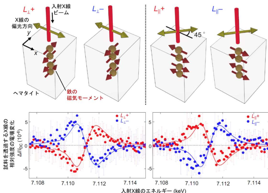
図1：(上) ヘマタイトにおける4種類の磁気ドメイン状態と実験配置の模式図。(下) 各磁気ドメイン状態における電場で誘起されるX線透過率の相対変化スペクトル。ピーク振幅200 Vの交流電圧を印加した条件下で測定された。実線は \text{Fe}^{3+} イオンと \text{O}^{2-} イオンの相対変位を5 fmとしたときの第一原理計算による数値シミュレーションの結果を表す。
