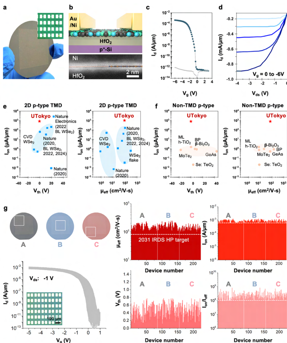
図2：ウエハスケールのBCNトランジスタアレイと電気特性
