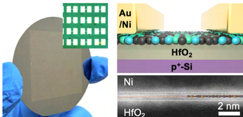
2 インチウエハー上に作製した単層 BCN トランジスタアレイと素子構造
