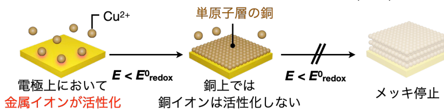
図 1：アンダーポテンシャル電解重合（本研究、UPEP）とアンダーポテンシャル析出（過去の研究）の比較
