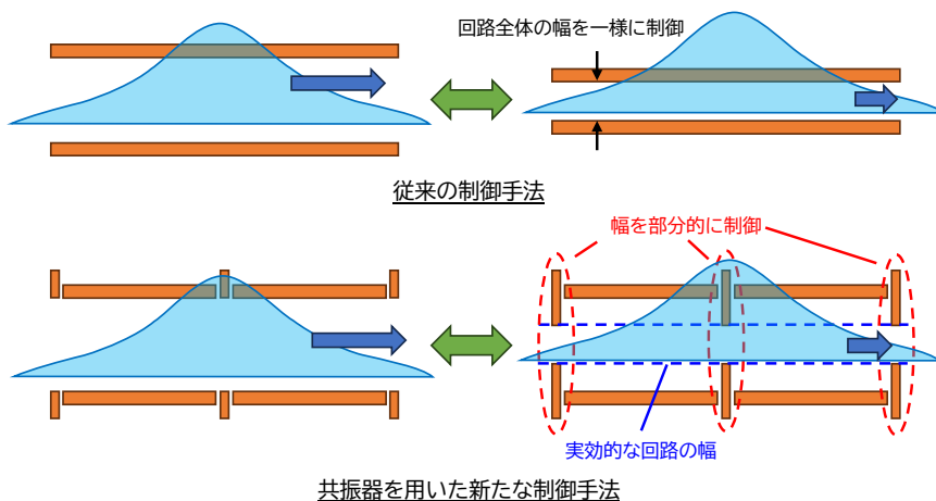
図 1: 従来の固有状態制御手法と本研究で開発した新手法の比較。従来の手法では、プラズモン波束(水色)が通過する回路全体の幅を一様に制御していました。回路の幅が広いとプラズモン波束の速度は大きく、幅が狭いと小さくなります。共振器を用いた新たな手法では、部分的に幅を制御することで、回路全体の実効的な幅を狭くする効果を得ることができます。
