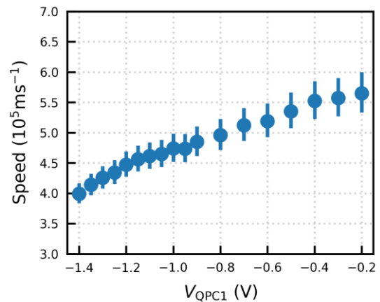
図 2: QPC の閉じ込め幅に依存したプラズモン波束の速度。横軸に沿った QPC における回路幅の部分的な変調によって、プラズモン波束の速度が制御される様子を示している。
