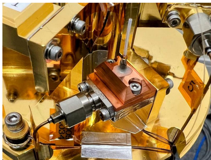
図 2：東京大学と NICT が共同開発した超伝導光子検出器
