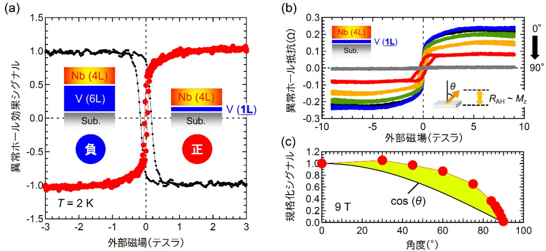
図 2: (a) NbSe 2 / V 5 Se 8 磁性 vdW ヘテロ構造の異常ホール効果。V 5 Se 8 が十分に厚いときは負の異常ホール効果（黒いデータ）を示すが、V 5 Se 8 を単層極限まで薄くすると正の異常ホール効果（赤いデータ）が出現する。(b) 正の異常ホール効果を示す試料に対して測定した異常ホール効果の外部磁場角度依存性。外部磁場を面直（0°）から面内（90°）に傾けると、異常ホール効果のシグナルは全体的に減少する。(c) 磁場 9 T におけるシグナルの角度依存性。一般に外部磁場を面内に傾けるとシグナルは \cos\theta に従って単調に減少するが、この試料では一度「増大」してから減少する極めて異常な振る舞いが観測された。この振る舞いは計算でよく再現され、NbSe 2 がフェロバレー強磁性を形成していることを示す直接的な証拠となっている。
