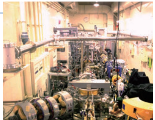
極短パルスの電子線を発生するLINAC施設
