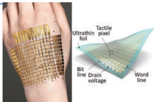
世界でもっとも軽く薄く柔らかい電子回路でできたタッチセンサ
