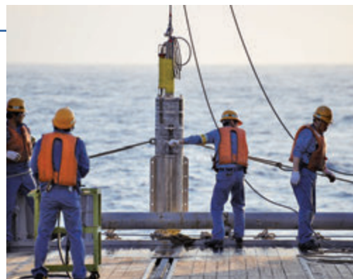
南鳥島レアアース泥のピストンコアラールによる探査
