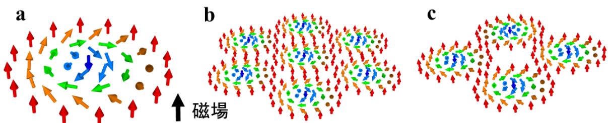
図1：スキルミオンおよびスキルミオン格子の模式図
