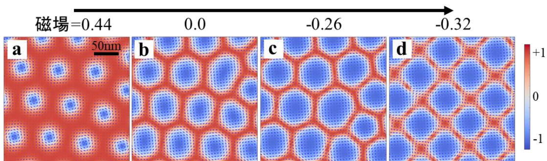
図 3 : 計算機シミュレーションによって得られた磁気構造
