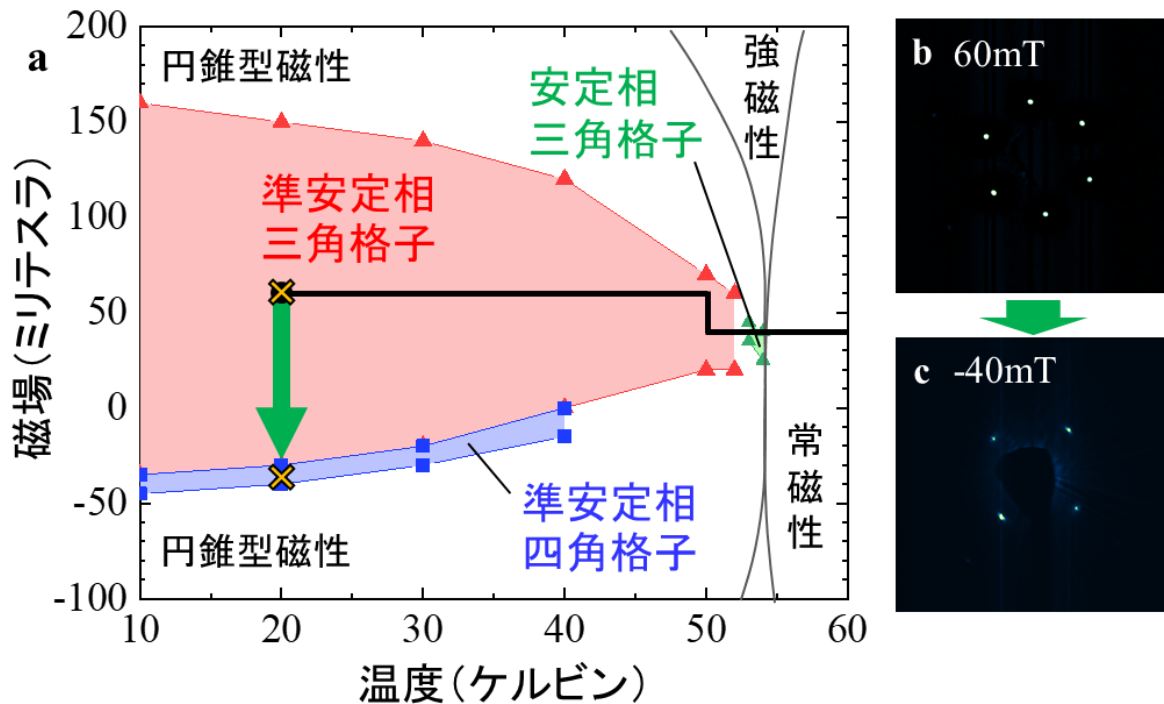
図 2 : \text{Cu}_2\text{OSeO}_3 の準安定状態図と軟エックス線散乱パターン
