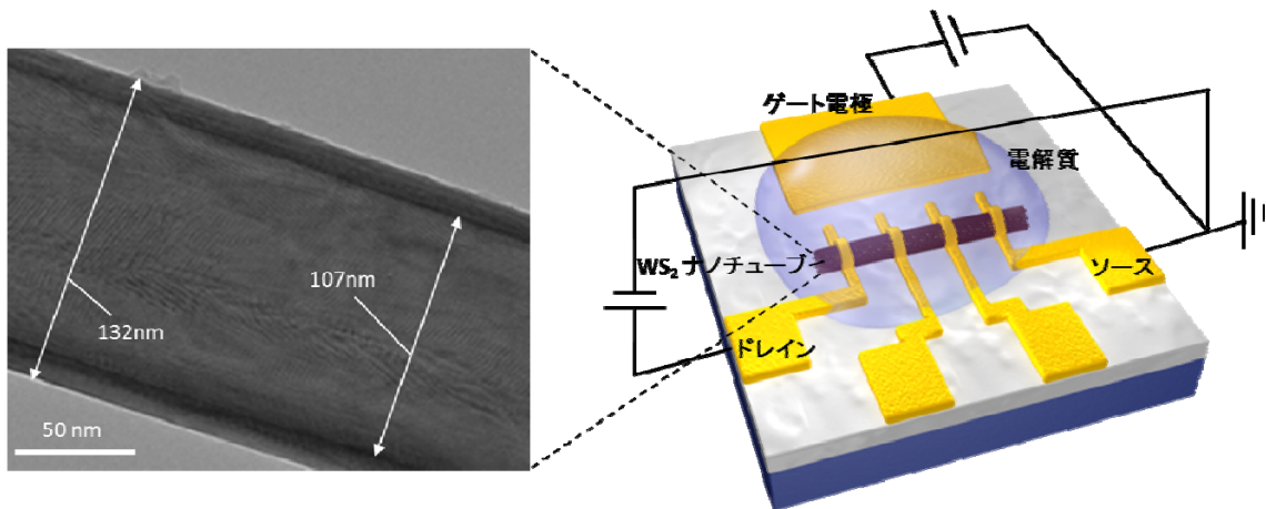
図1. 多層二硫化タングステン( WS_2 )ナノチューブの透過型電子顕微写真とデバイスの模式図 試料は直径 100 ナノメートル程度の多層ナノチューブである。正のゲート電圧を印加することで、 WS_2 ナノチューブの表面および層間に正イオンが集積し、試料中に電子が蓄積される。
