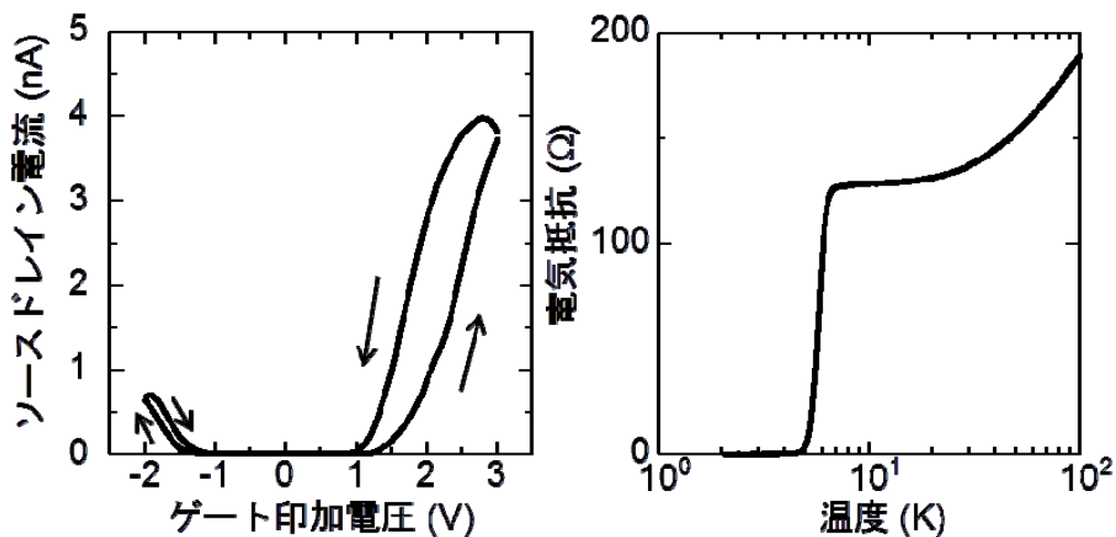
図2. WS_2 ナノチューブのトランジスタ動作と超伝導の発現 ゲート印加電圧が正負どちらの領域でも金属的挙動が実現でき、電子を多量に蓄積した領域では 5.8 ケルビン（マイナス 267.4℃）以下で電気抵抗がゼロになる超伝導が発現している。
